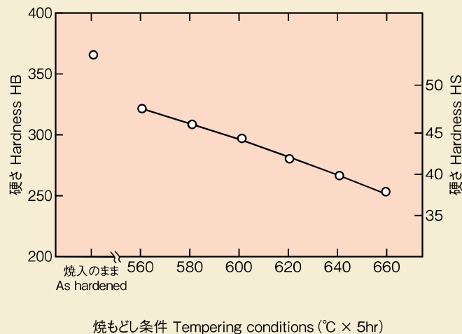
図1 焼もどし硬さ曲線 Fig. 1 Tempered hardness curve
