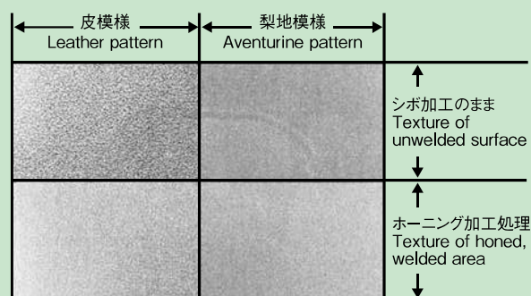
写真2 シボ加工模様 Photo. 2 Texture patterns
