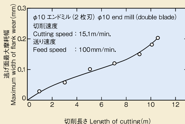
図3 被削性 Fig. 3 Machinability
