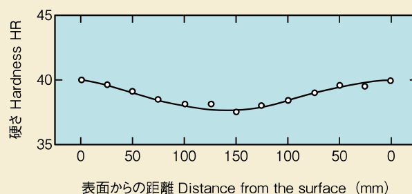
図2 断面硬さ分布 Fig. 2 Sectional hardness distribution
